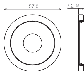
ROSETA REDONDA DUPLA RETA - CÓD. 095
