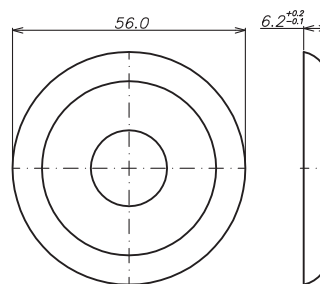
Roseta Redonda Chanfrada CÓD. 088
