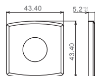
ROSETA ABAULADA CÓD. 081
