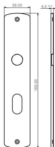
ESPELHO RENTAGULAR CÓD.226
