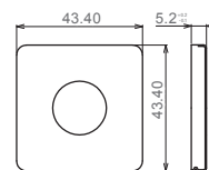
ROSETA QUADRADA PEQUENA CÓD. 080
